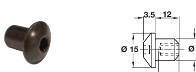
F M6 sleeve nut
