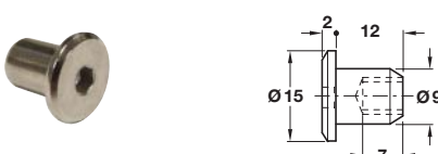
E M6 Sleeve nut
