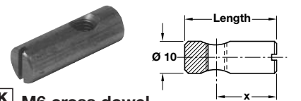
K M6 cross dowel
