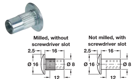
I M6 sleeve nut
