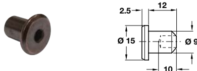
D M6 sleeve nut
